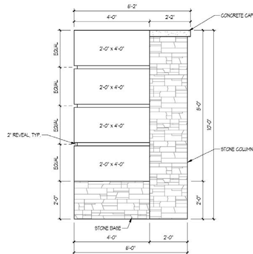
2 MONUMENT SIGN SCALE: 1/2" = 1'-0"
