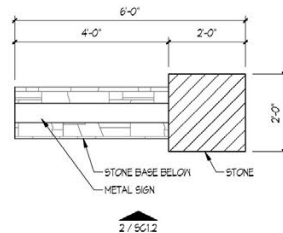
1 MONUMENT SIGN SCALE: 1/2" = 1'-0"
